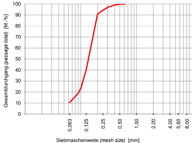
Mittlere Sieblinie (average grading curve)
